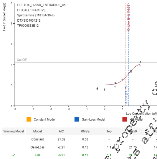
Figure CA 5.8.3/09-21: CEETOX_H295R ESTRADIOL_up
