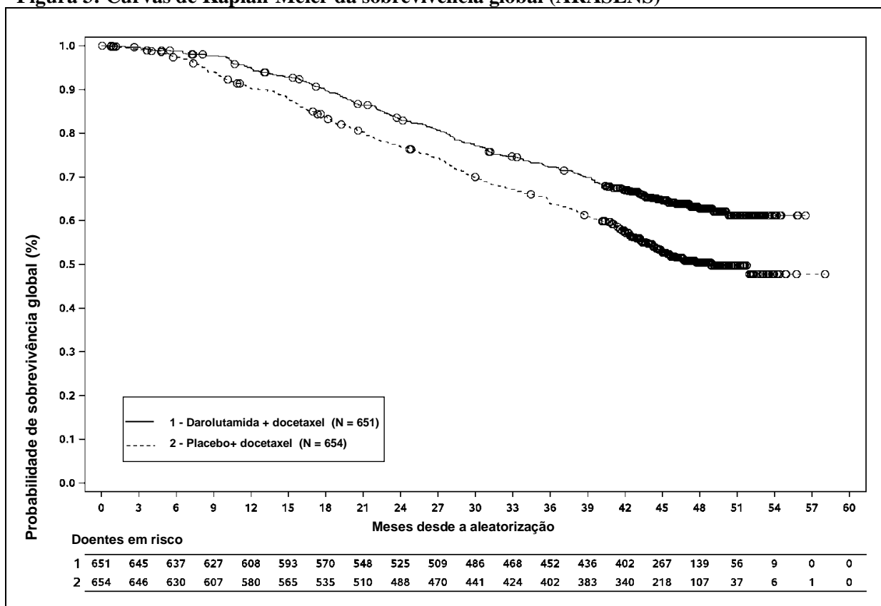
Figura 3: Curvas de Kaplan-Meier da sobrevivência global (ARASENS) a
